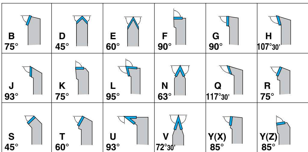
Rodzaj noża / Toolholder type 3
