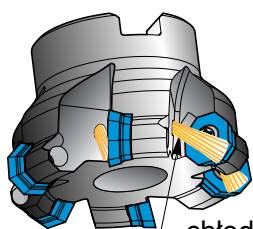
chłodzenie coolant
